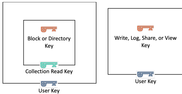
Key Wrapping
